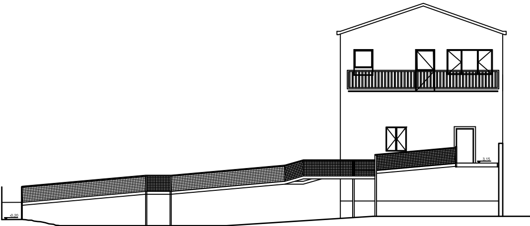
ELEVACION PATIO CON PASARELA 1:50
