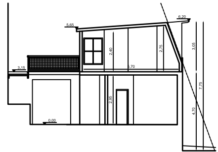
CORTE B 1:50
