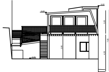
ELEVACION PATIO 1:50
