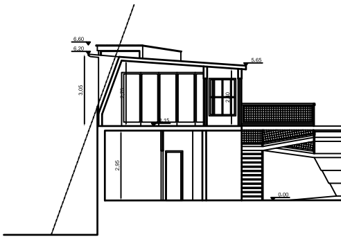
ELEVACION PATIO INTERIOR 1:50
