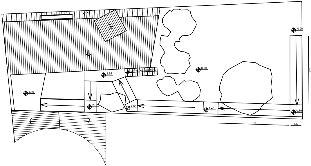
PLANTA TECHO 1:50
