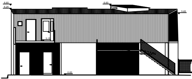
ELEVACION PATIO INTERIOR 1:50
