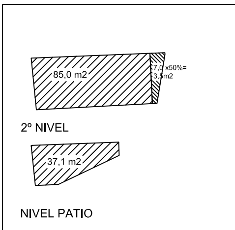
PLANO SUPERFICIE 1:100
