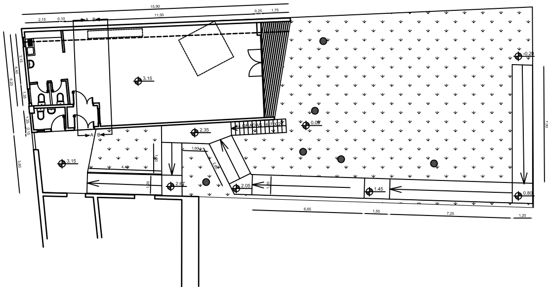
PLANTA NIVEL SALA 1:50
